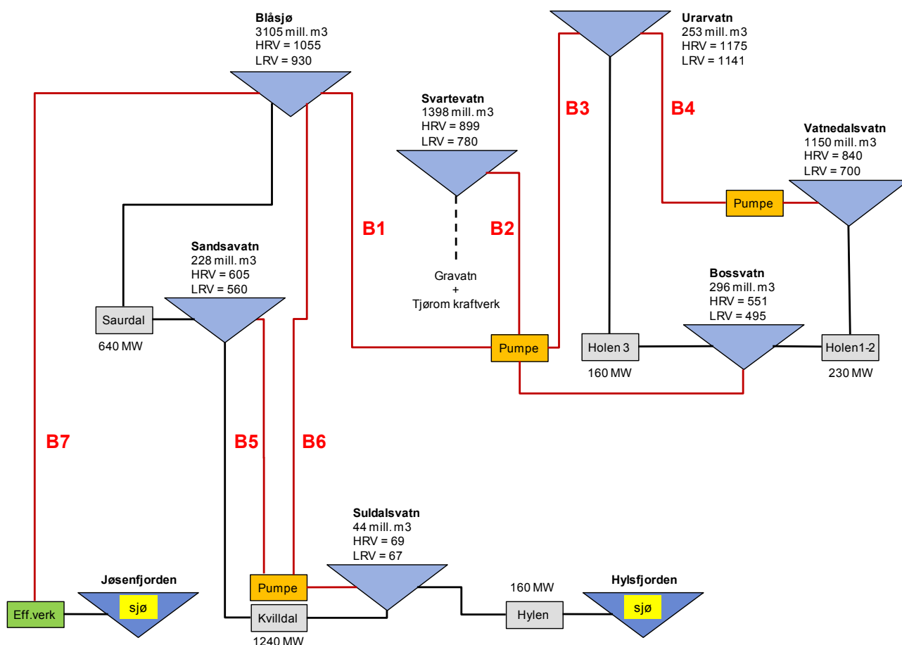
Figur 2.4: Case Blåsjø – Svartevatn – Otramagasinene.
